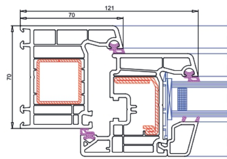
Sección lateral
